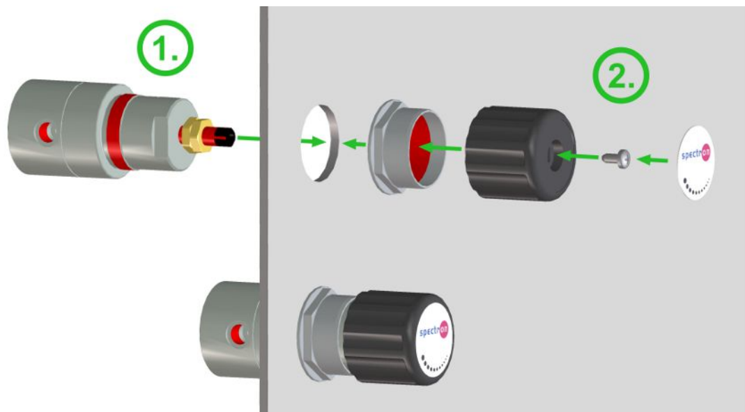
3: Montaggio a pannello riduttore di pressione serie 50
