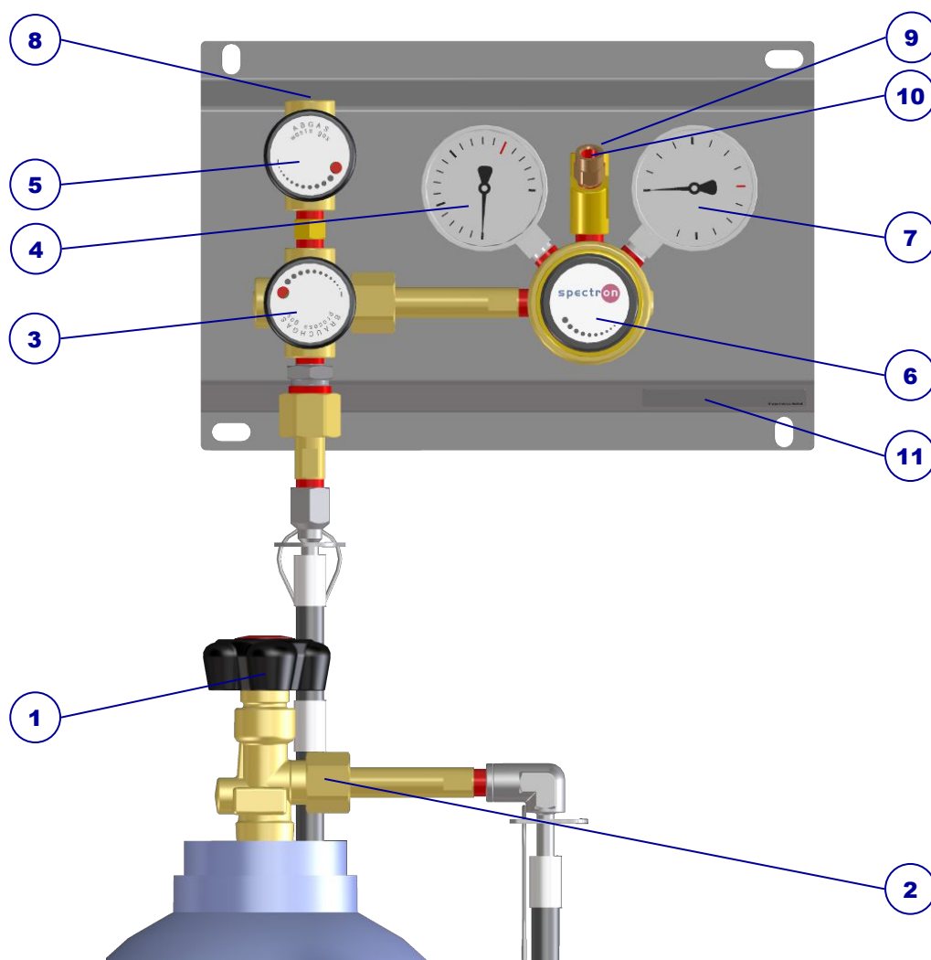
1: Design centrale di decompressione BT2000-1
