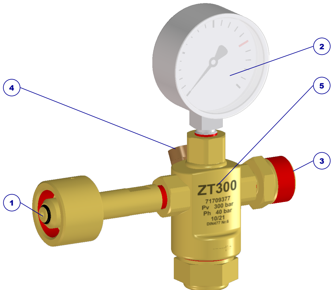
Abb. 1: Aufbau Druckregler ZT300
