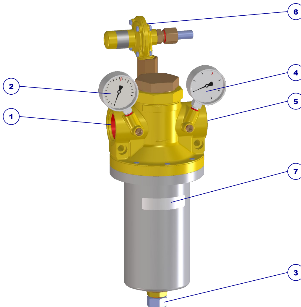
Abb. 1: Aufbau Druckregler U47AC
