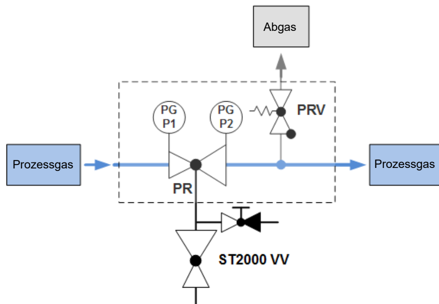
Abb. 2: Schema U43AC
