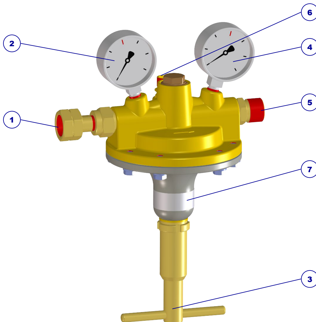
Abb. 1: Aufbau Druckregler U23AC
