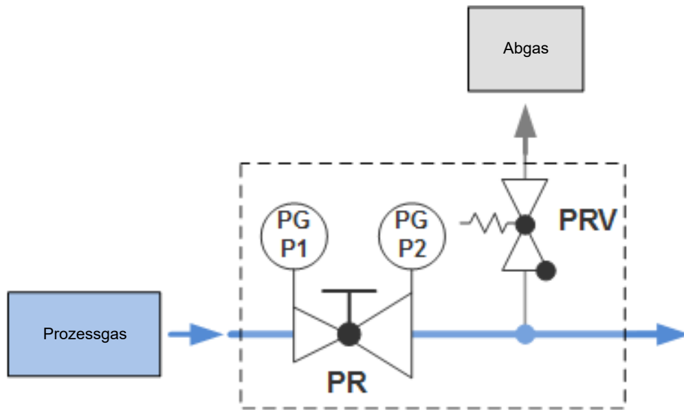
Abb. 2: Schema U23AC
