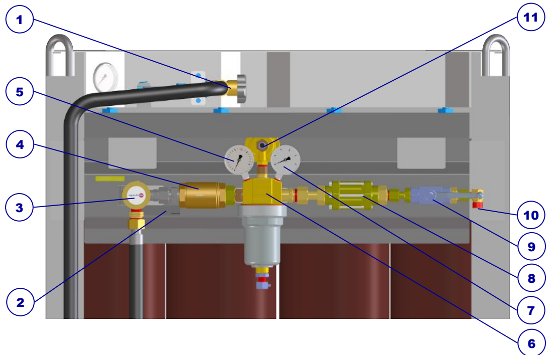
Abb. 1: Aufbau MU13AC
