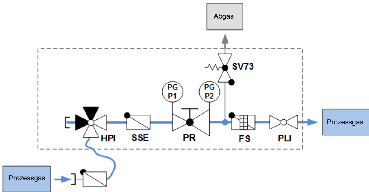
Abb. 2: Schema MU13AC–SSE
