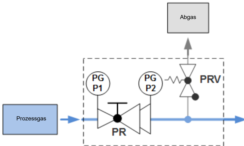
Abb. 2: Schema M53
