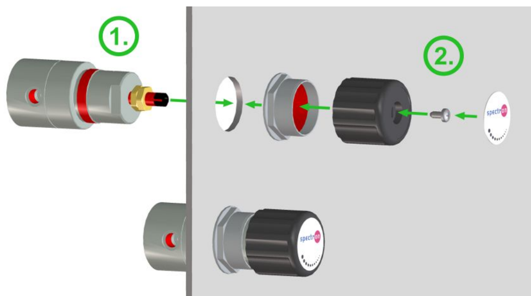
Abb. 3: Tafeleinbau 50er-Panel-Druckregler
