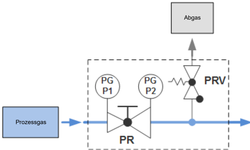
Abb. 2: Schema M51
