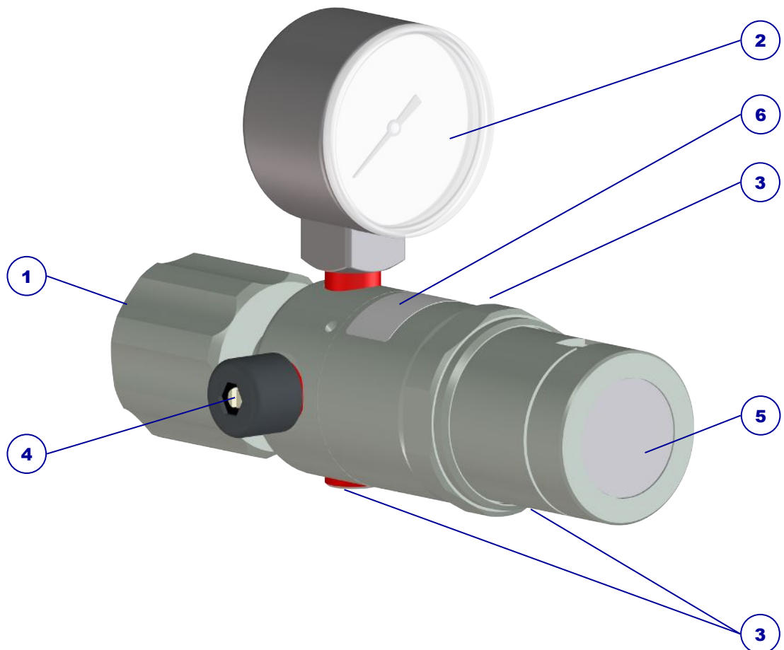
Abb. 1: Aufbau Druckregler FM35-L
