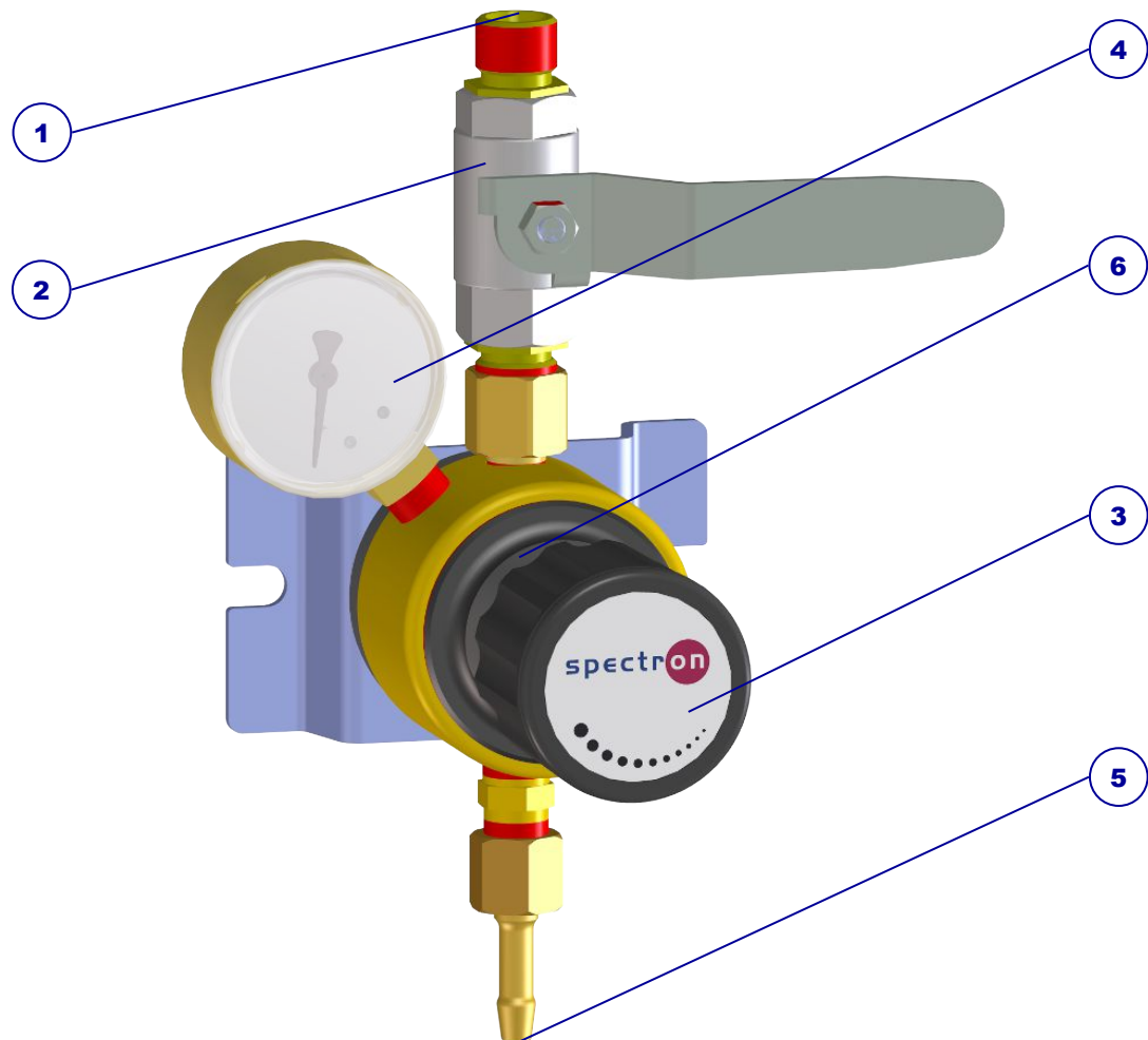
Abb. 1: Aufbau Entnahmestelle ET65-BV
