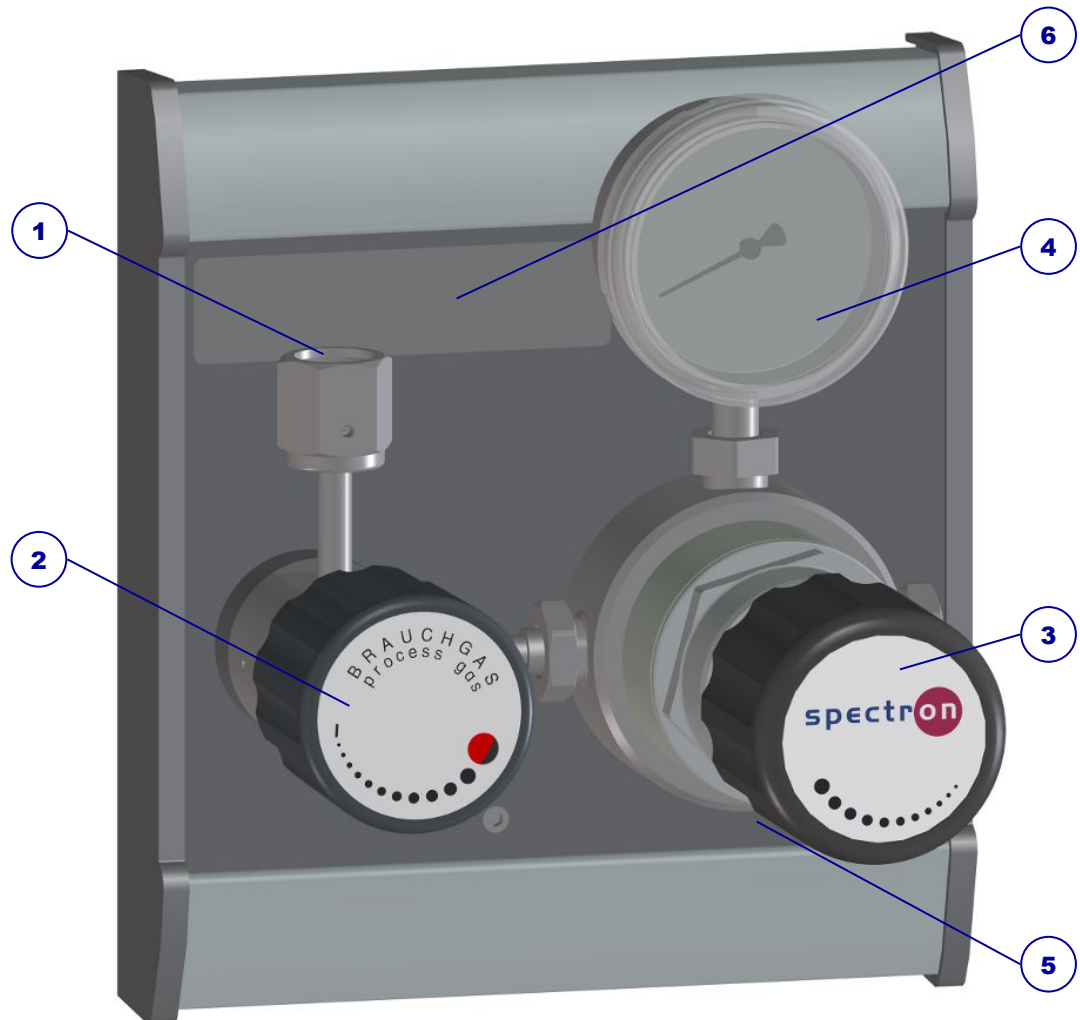
Abb. 1: Aufbau
