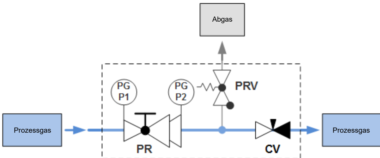
Abb. 2: Schema CRF62
