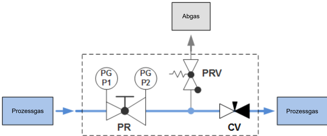
Abb. 2: Schema CRF61
