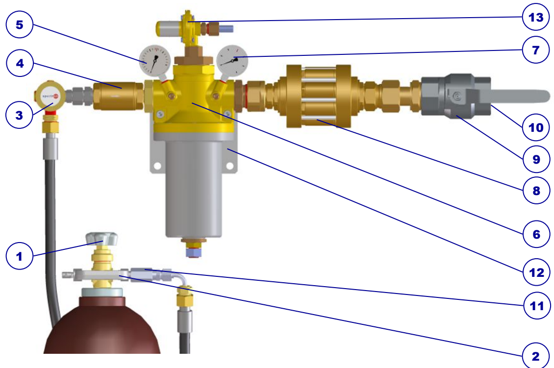
Abb. 1: Aufbau BU47AC-SSE
