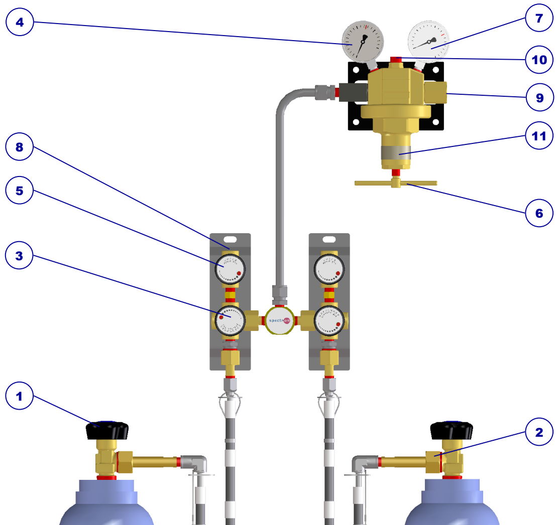
Abb. 1: Aufbau Entspannungsstation BU15-2
