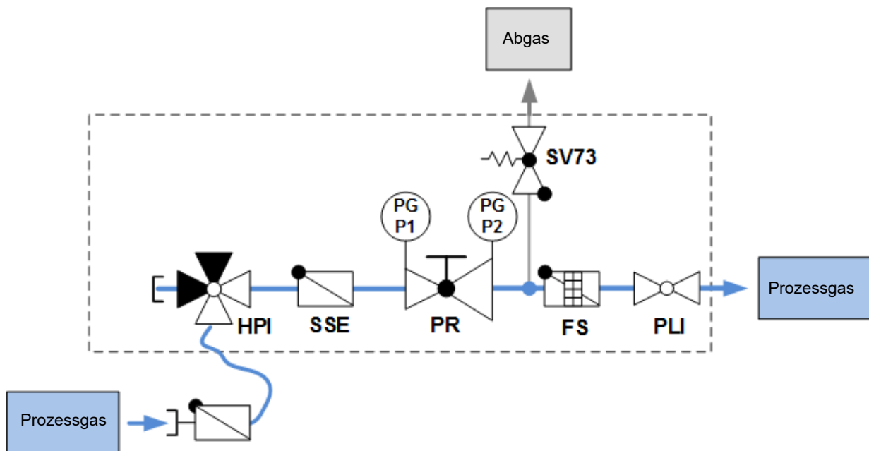
Abb. 2: Schema BU13AC–SSE
