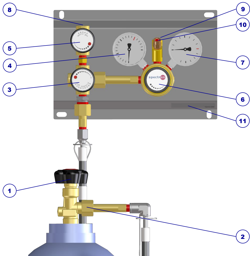
Abb. 1: Aufbau Entspannungsstation BT2000-1
