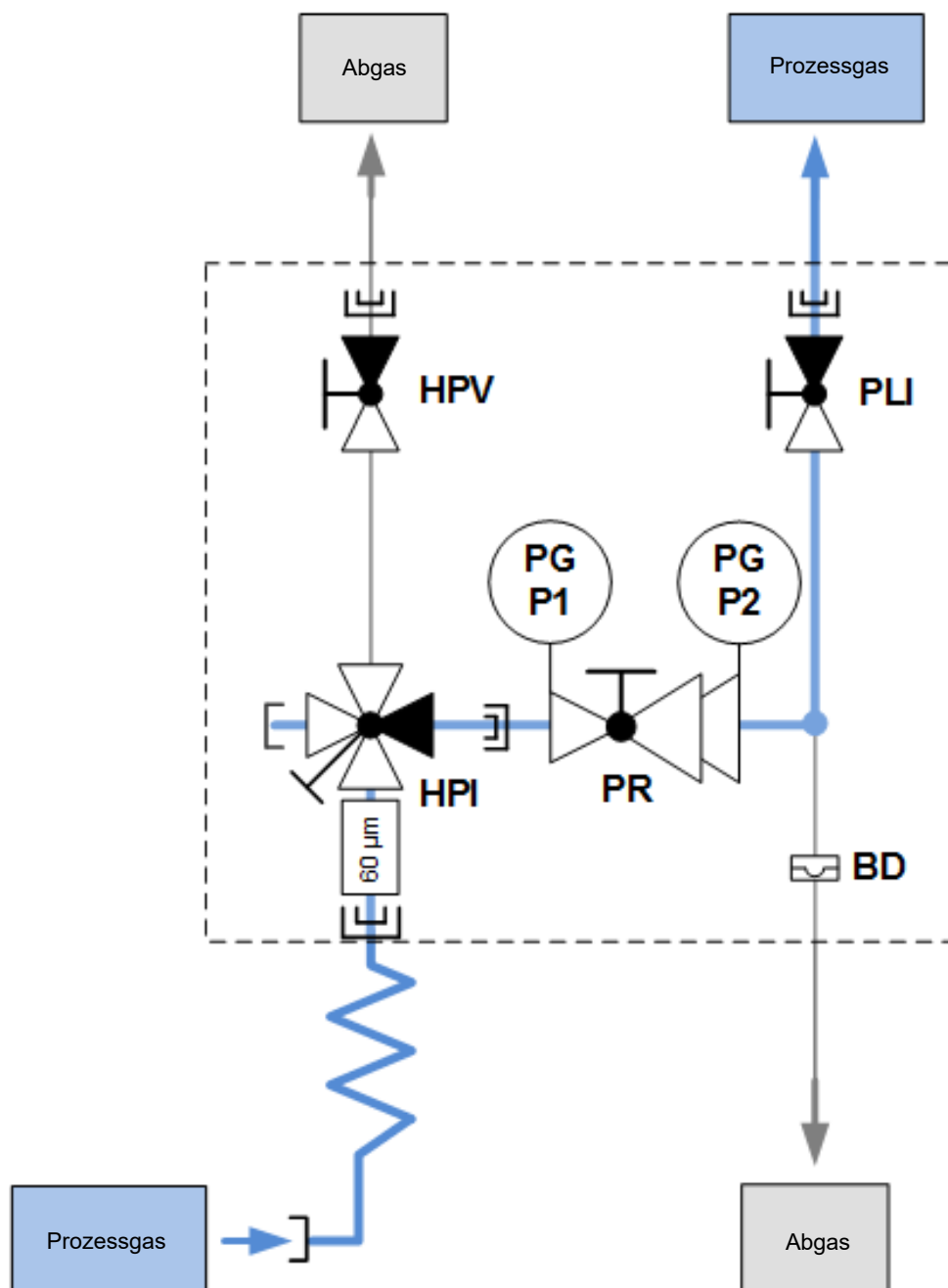
Abb. 2: Schema BE56-1-VCR
