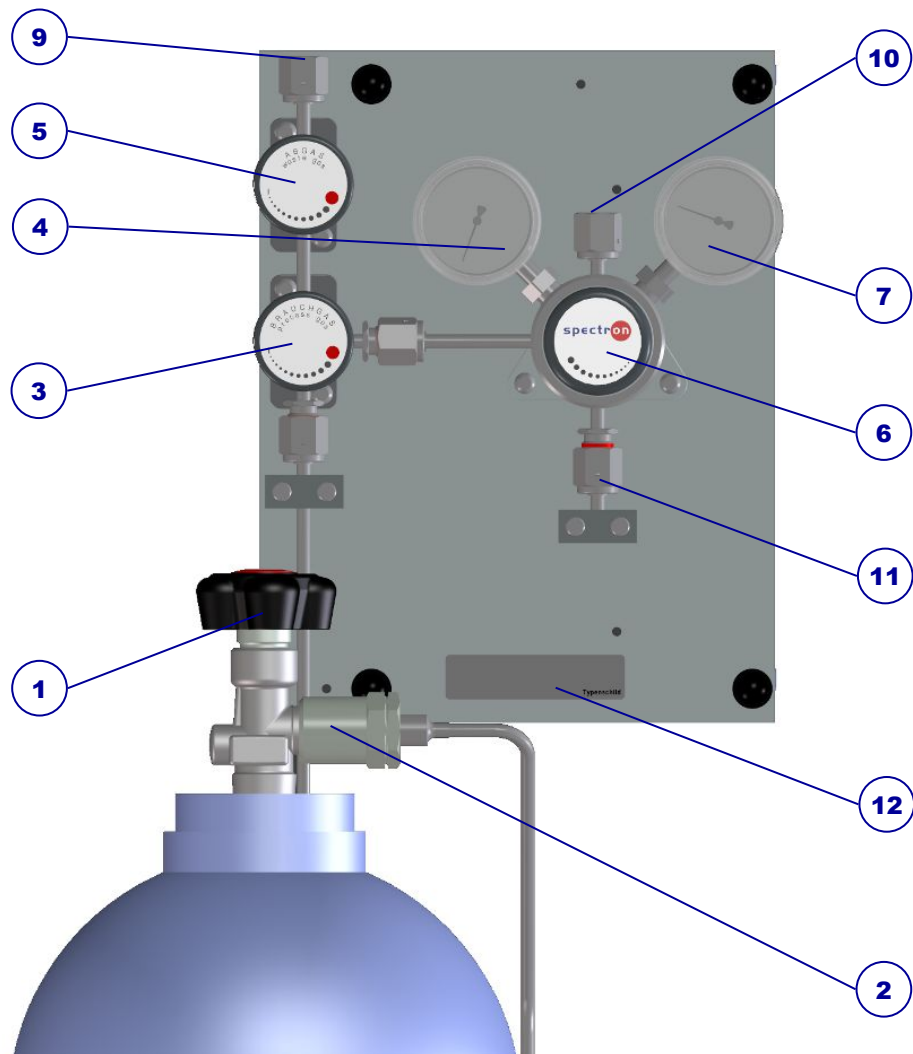
Abb. 1: Aufbau Entspannungsstation BE56-1-VCR
