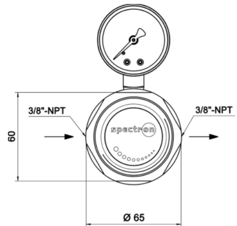
Hauptabmessungen
