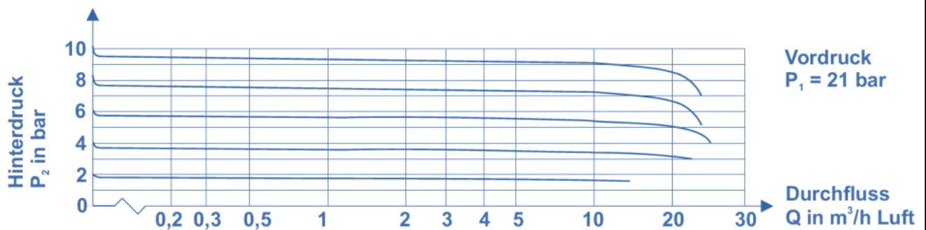
Durchflusskennlinien BM56-1
