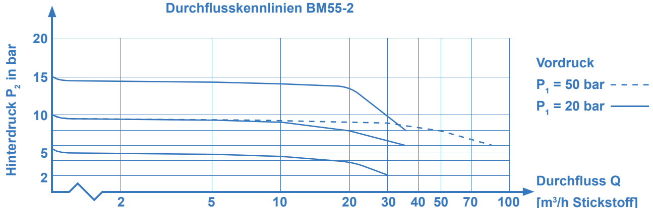
Durchflusskennlinien BM55-2
