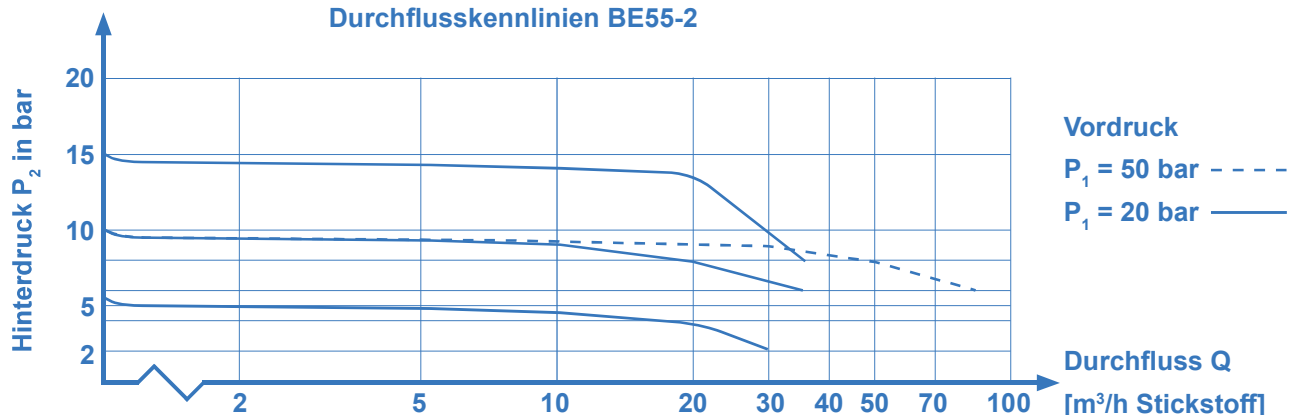
Durchflusskennlinien BE55-2
