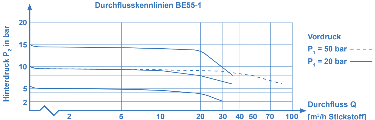
Durchflusskennlinien BE55-1
