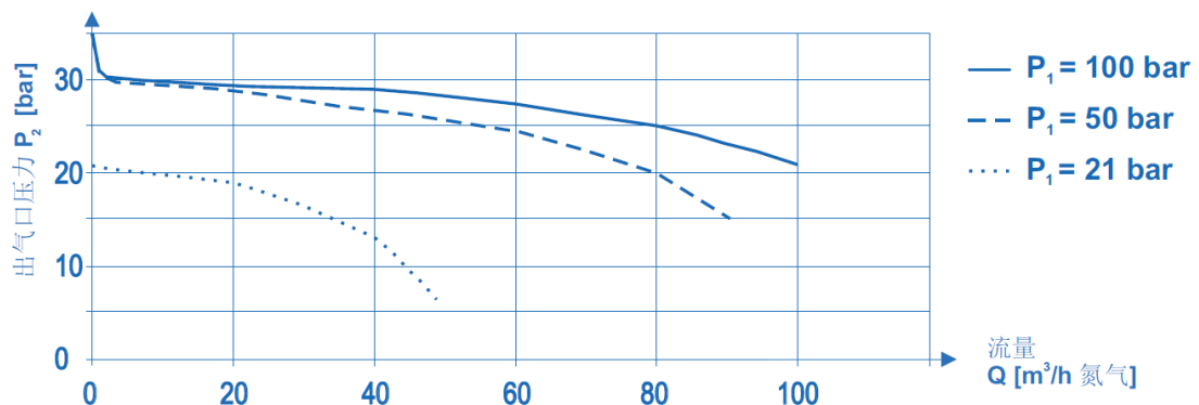
流量图
