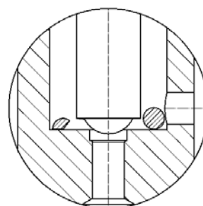
细节: 截止阀
