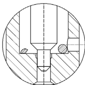
细节: 节流阀
