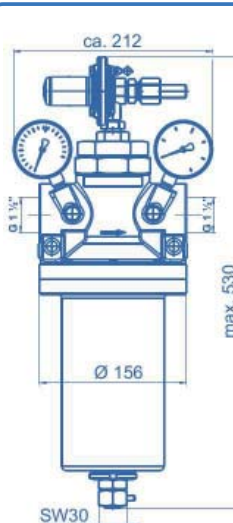
尺寸图
