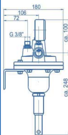
尺寸图
