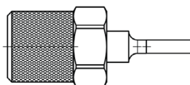
用于DIN 477 钢瓶阀的滚花接头(用于非腐蚀性气体)
