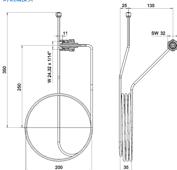
尺寸图: 配可手动连接 200 bar 的钢瓶接头
