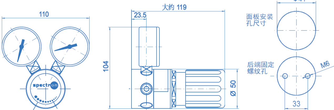
尺寸图 M51-6
