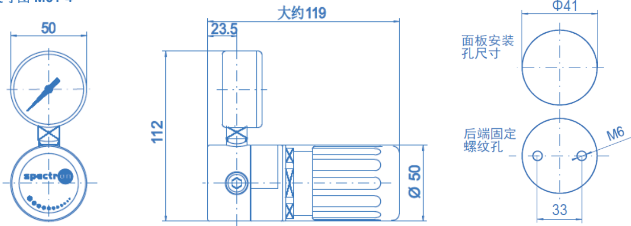
尺寸图 M51-4
