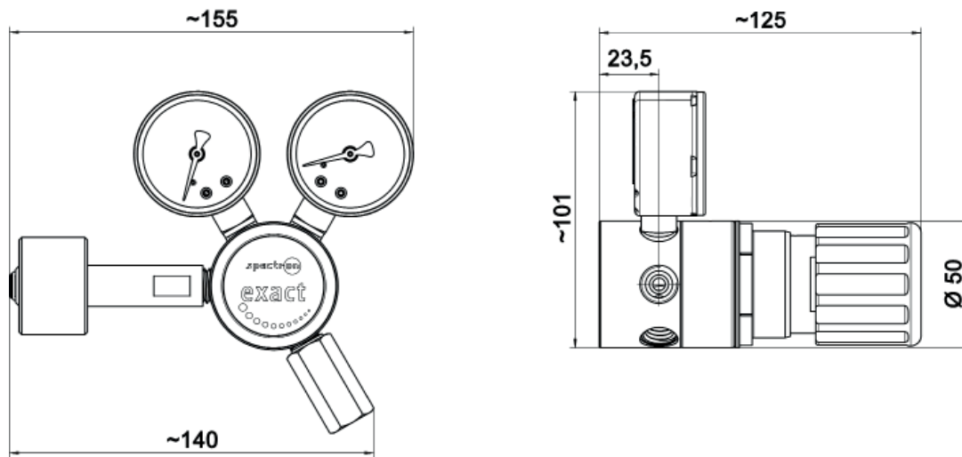
尺寸图 FE52
