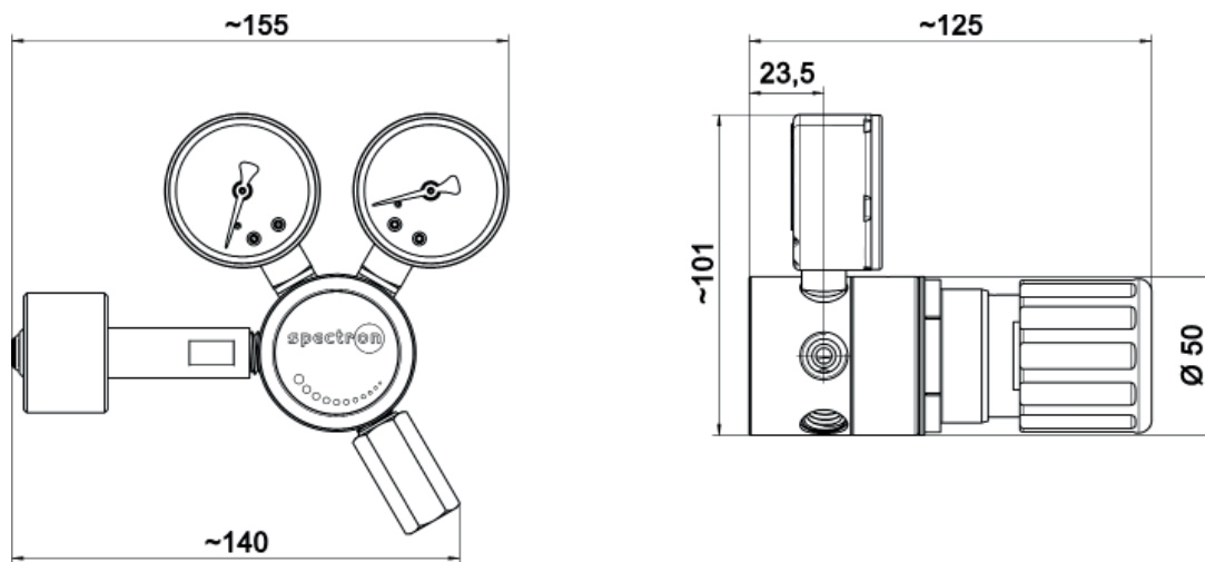
尺寸图 FE51
