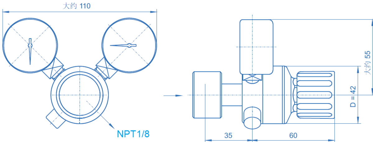
尺寸图 FE45
