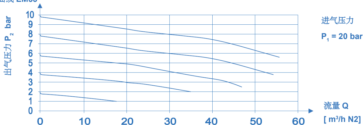
流量曲线 EM55
