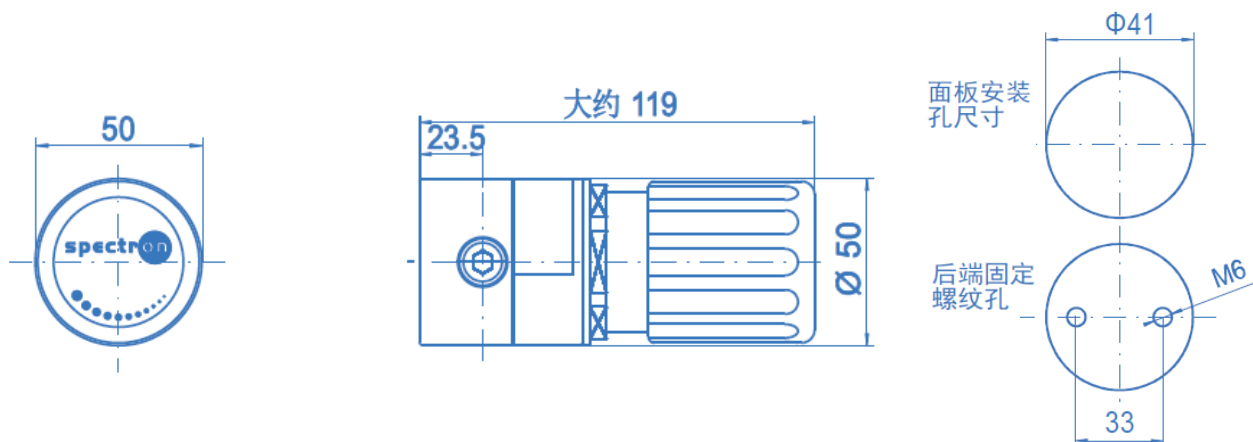
尺寸图 E52-2
