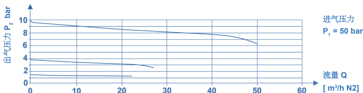
流量曲线 BM56-2U
