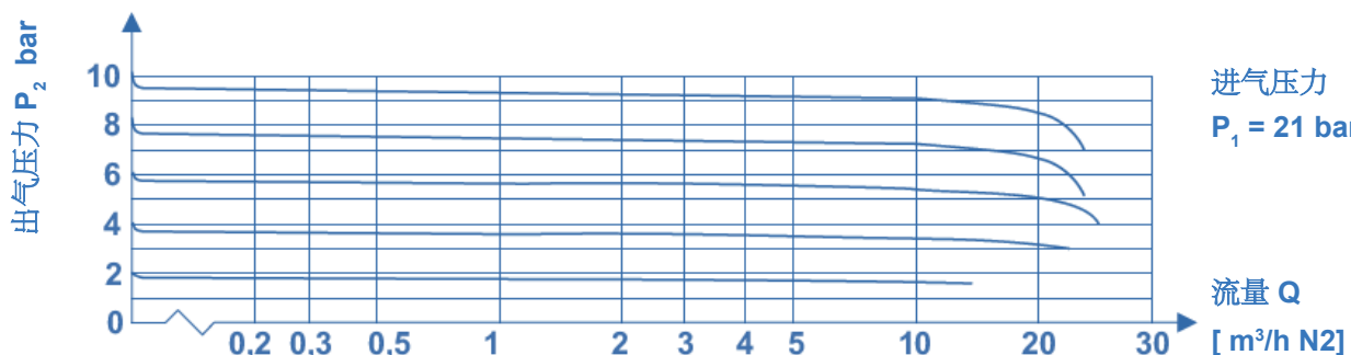
流量曲线 BM56-1
