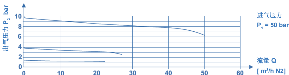
流量曲线 BE56-2U
