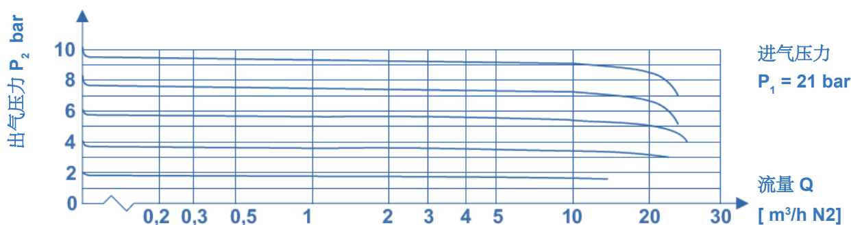
流量曲线 BE56-1
