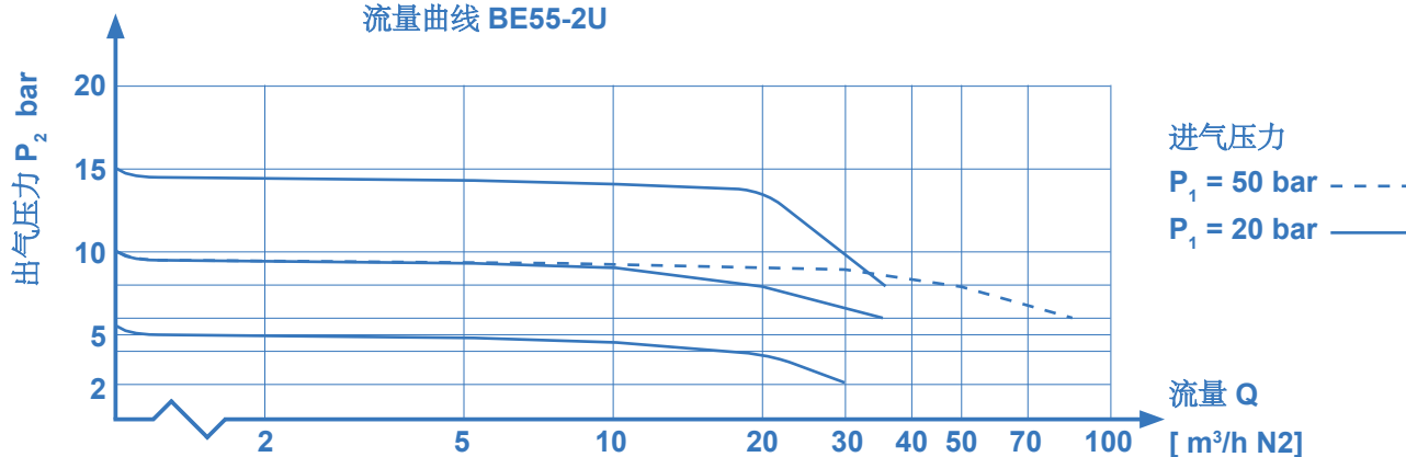
流量曲线 BE55-2U
