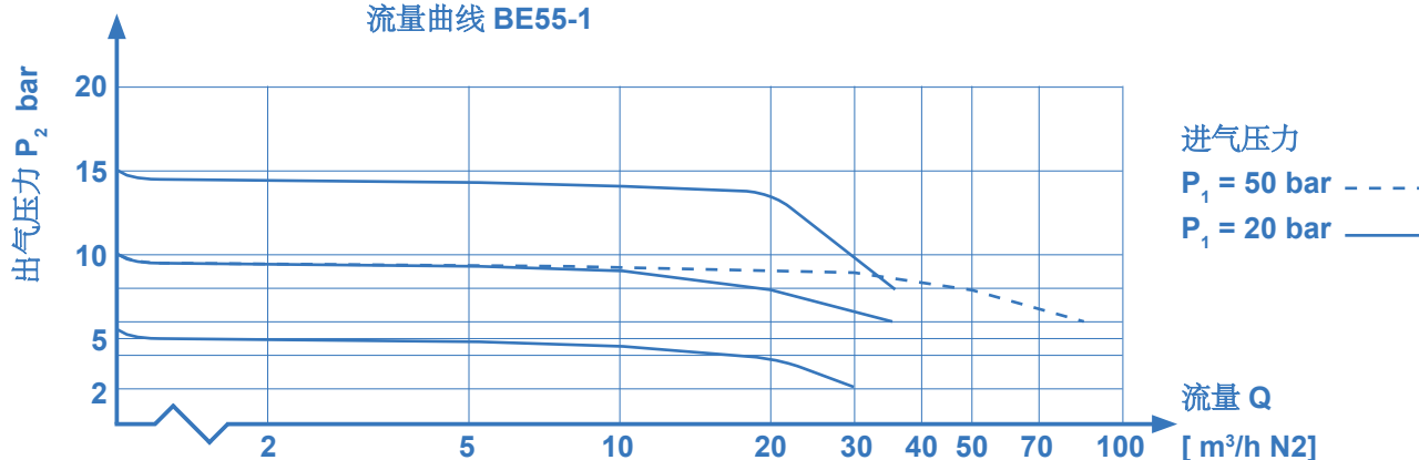
流量曲线 BE55-1
