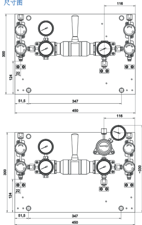
尺寸图
