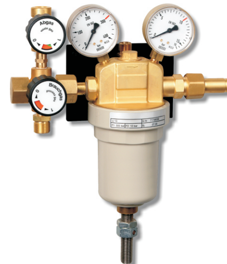
Rys. 1 Stacja rozprężania BU13 1x1
