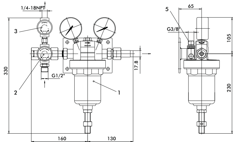
Rys.1 Stacja rozprężania U13 1x1 Dla 1 butli gazowej / wiązki
