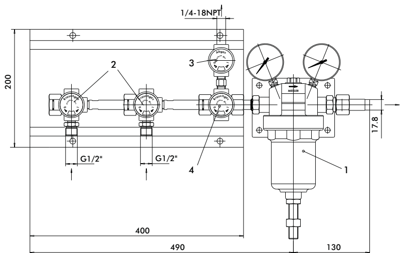
Rys.2 Stacja rozprężania U13 1x2 Dla 2 butli gazowych / wiązek
